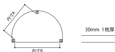
ST-183 半円形タイプ | スリット脚
